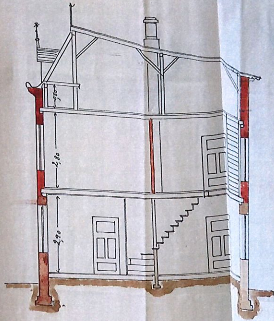
Querschnitt a-b
