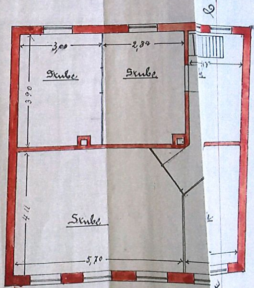
1. Etage
