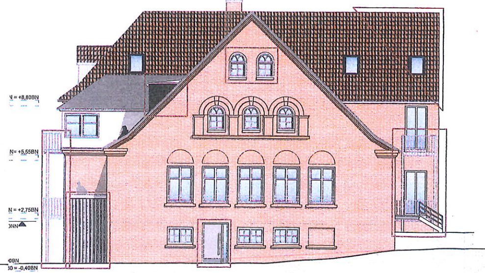
Ostansicht
